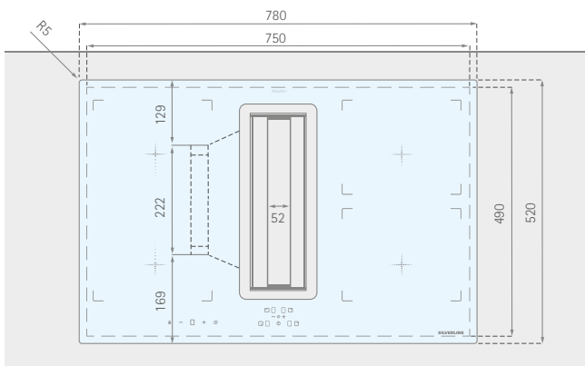
Kochfeld – Aufsatzmontage
