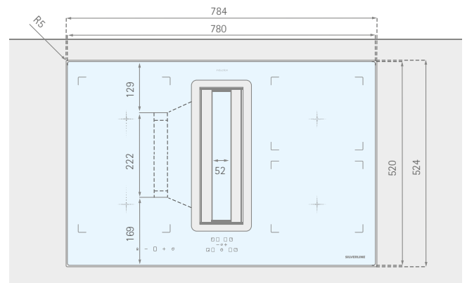
Kochfeld – flächenbündige Montage
