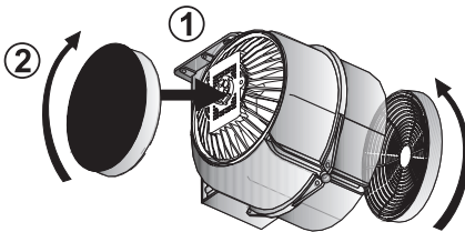
Abb.10: Einsetzen des Aktivkohlefilters AF110
