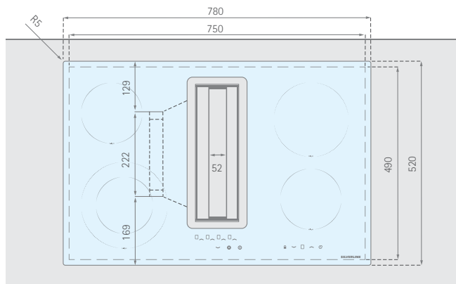
Kochfeld – Aufsatzmontage
